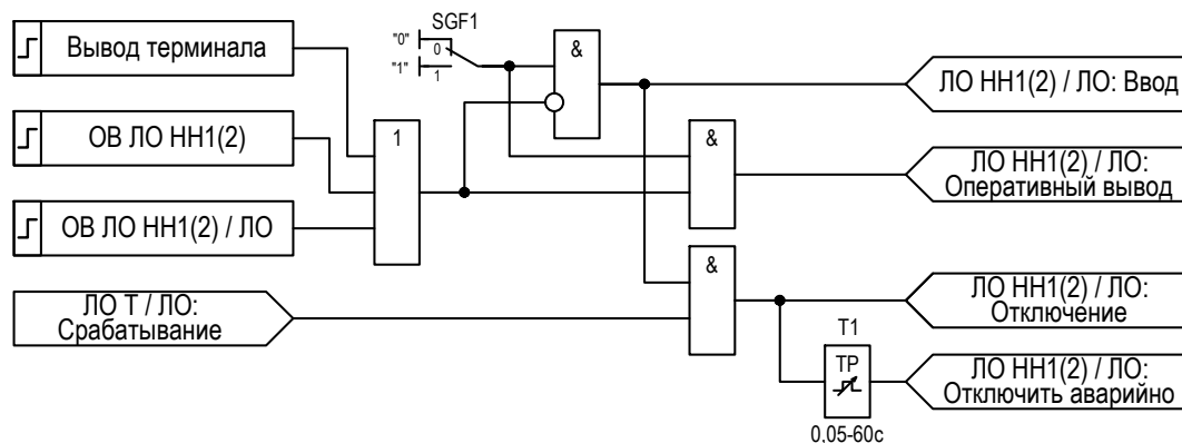
Рисунок 2.29 – Функциональная схема логики отключения выключателя
